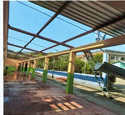
Foto 2: Mantenimiento de techo y estructura metálica
